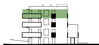
FASADE ØST
