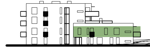
FASADE NORD
